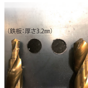
左: 4サイズドリル7.9-11-13 右: コバルトハイスドリル 13mm 4サイズなら約2倍の速さで穴あけ！ (当社比)
