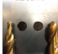
左:4サイズドリル7-9-11-13 右:コバルトハイスドリル 13mm 4サイズなら約2倍の速さで穴あけ! ※当社比
