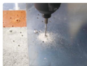
薄鉄板 (t1.6)+ブロック
